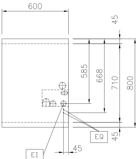
Boven aanzicht
