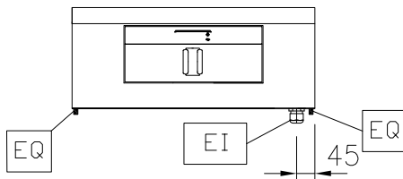
Front aanzicht
